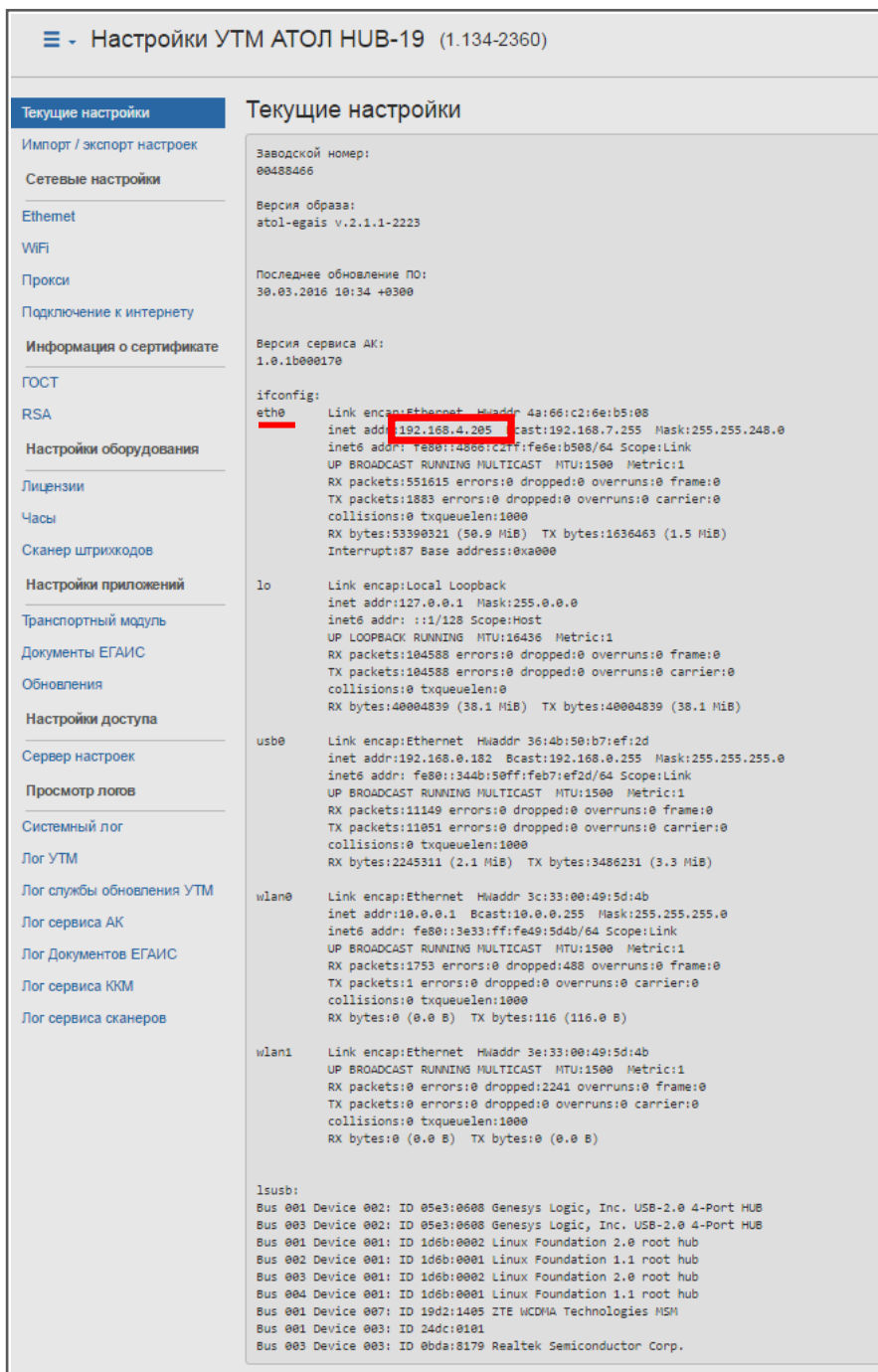
Рисунок 8. Текущие параметры. Динамический IP-адрес УТМ АТОЛ
