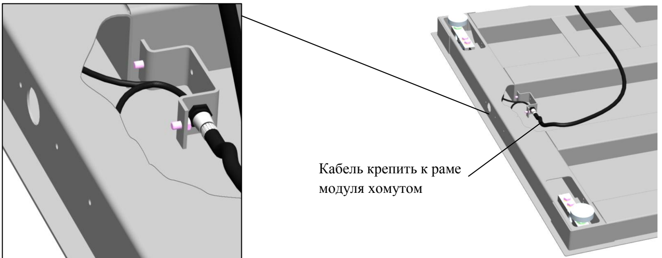
Рис. 2в. Монтаж разъема
