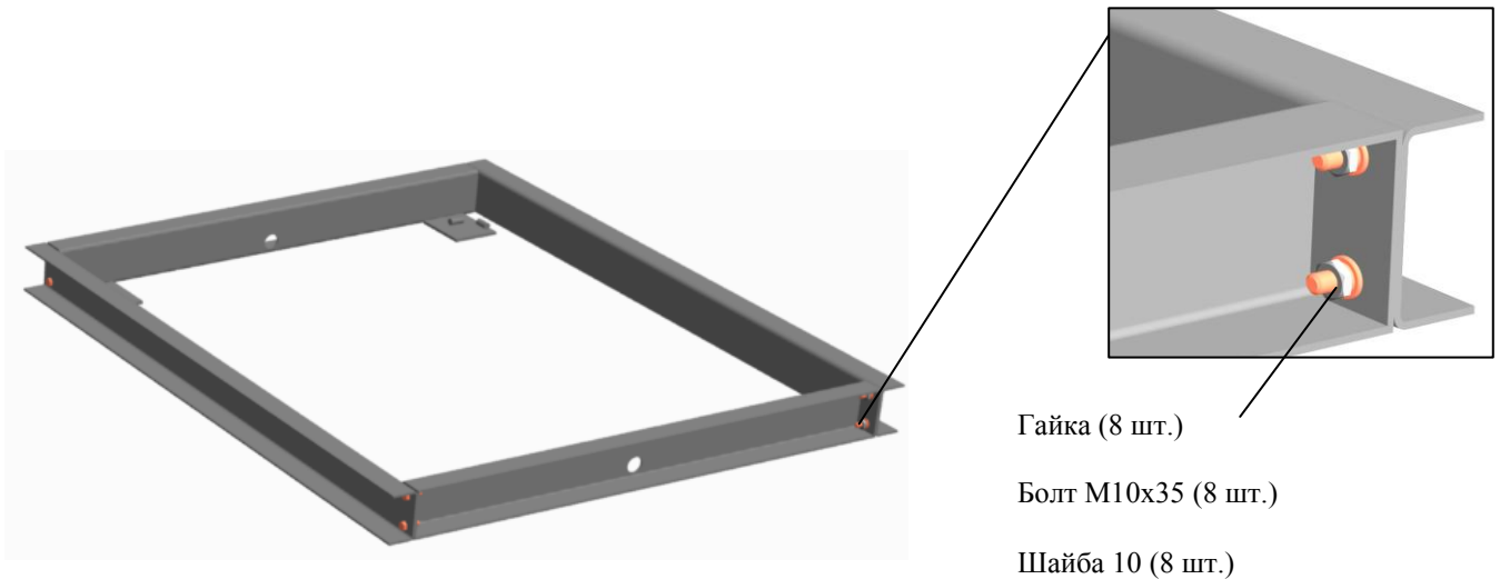
Рис.3. Сборка рамы
